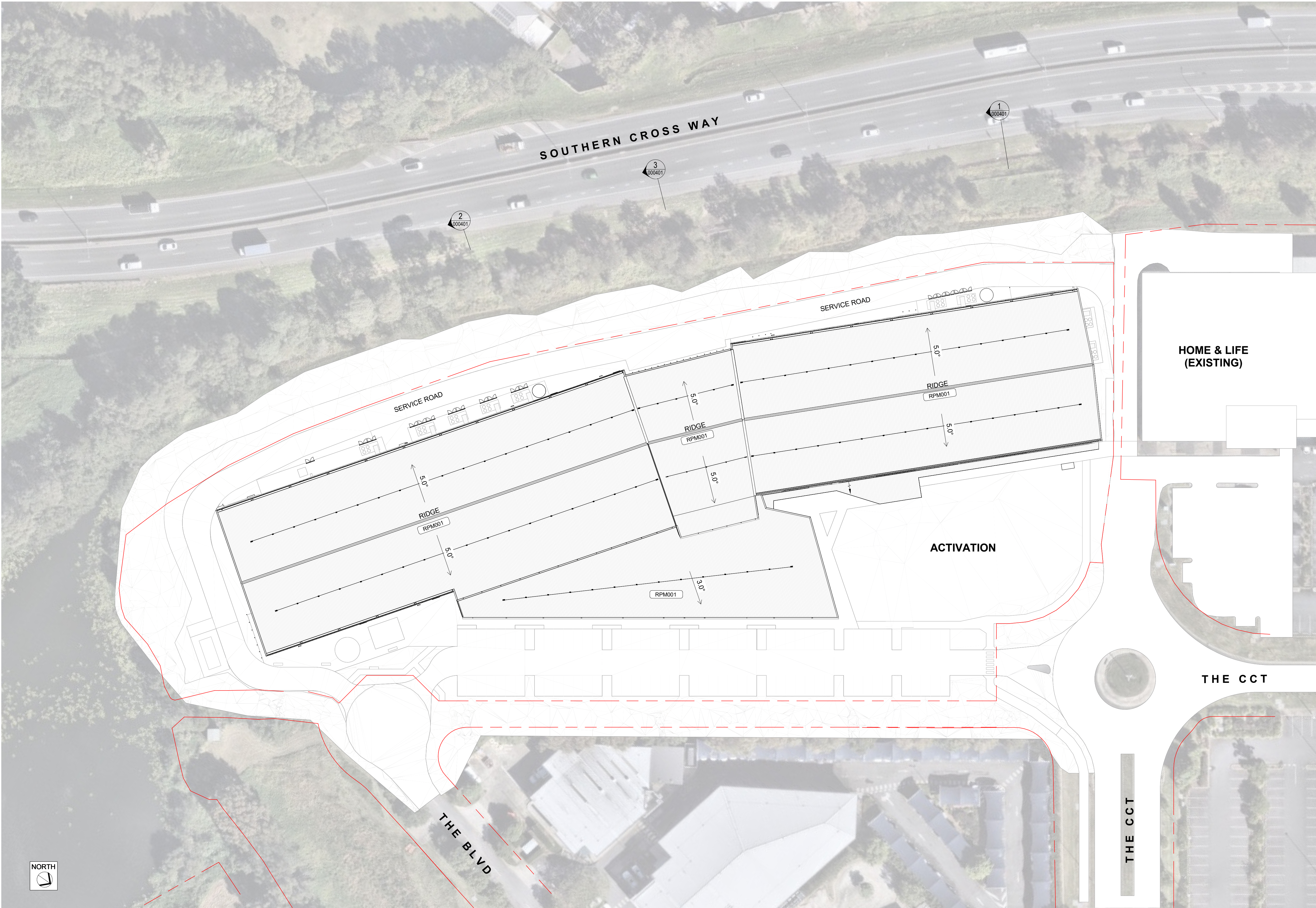
1 SITE PLAN 1 : 500
